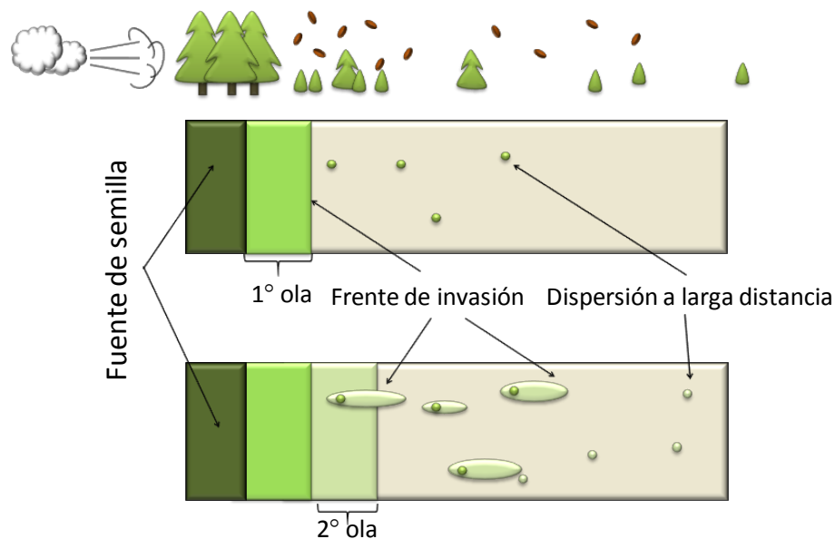
Figura 1. Diagrama del proceso de invasión generado por coníferas. Fuente: Langdon et al. 2010.
